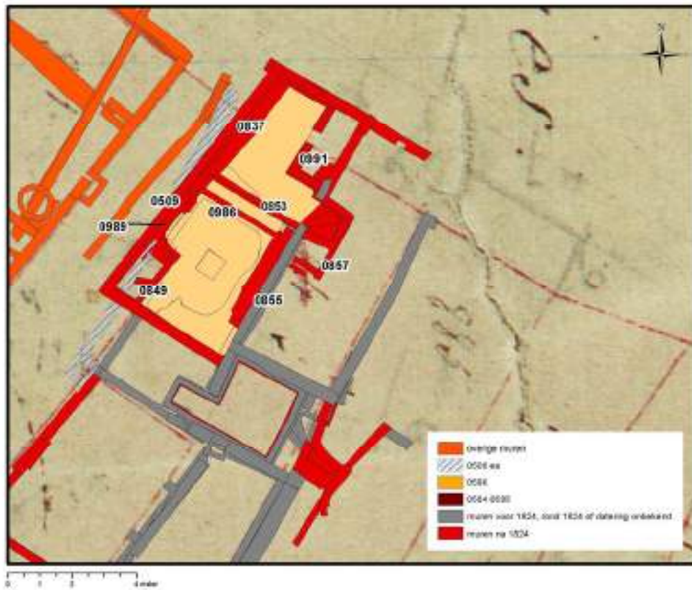
Figuur 3.3.7-70: na 1824, kelder aan de rooilijn
