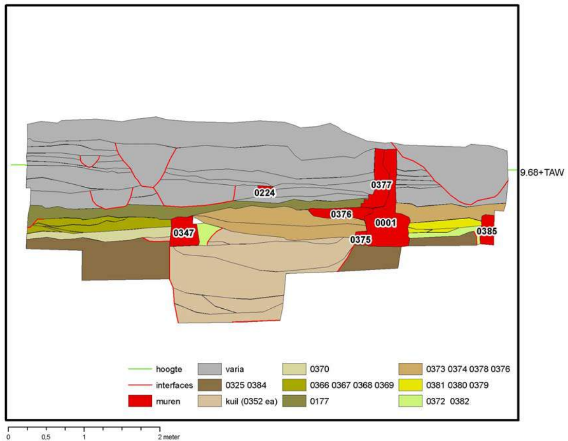
Figuur 3.3.5-79: profiel 2
