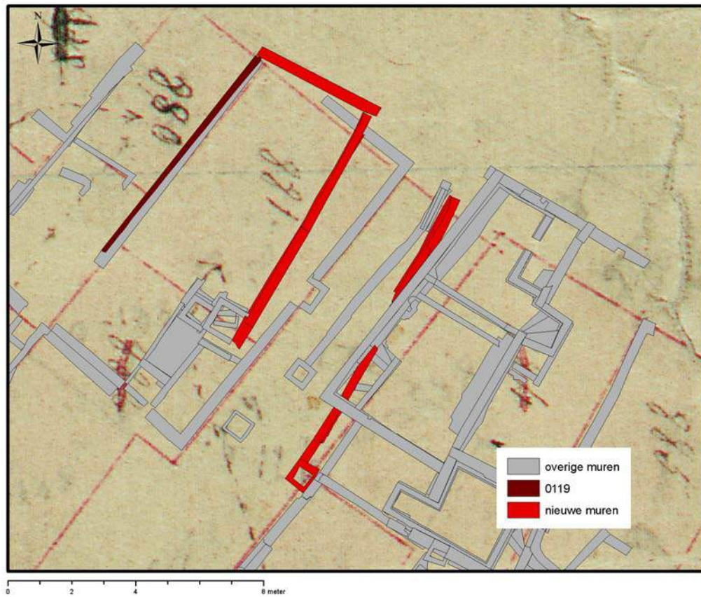
Figuur 3.3.7-31: muur 0119
