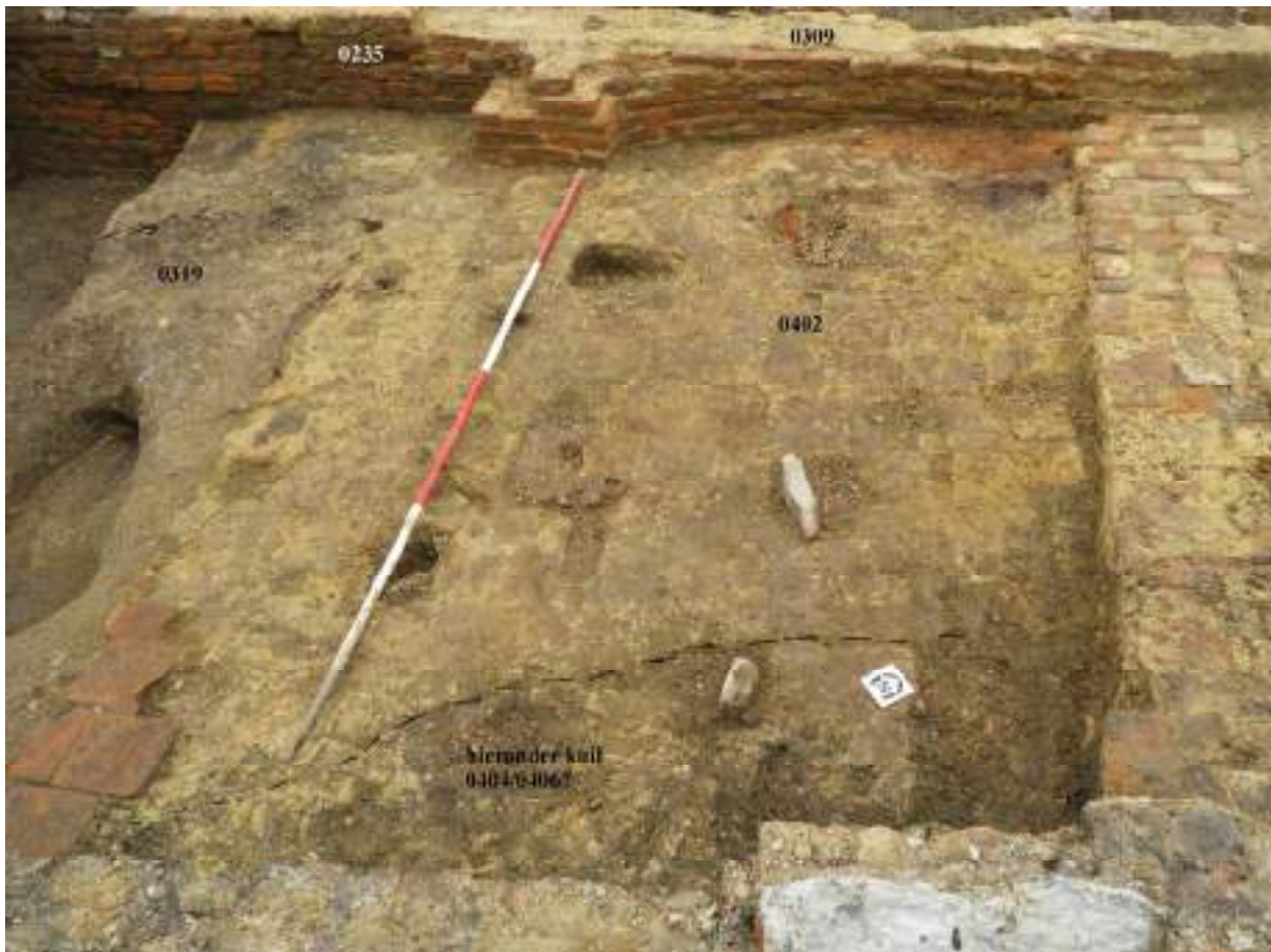
Figuur 3.3.5-41: vloer 0402
