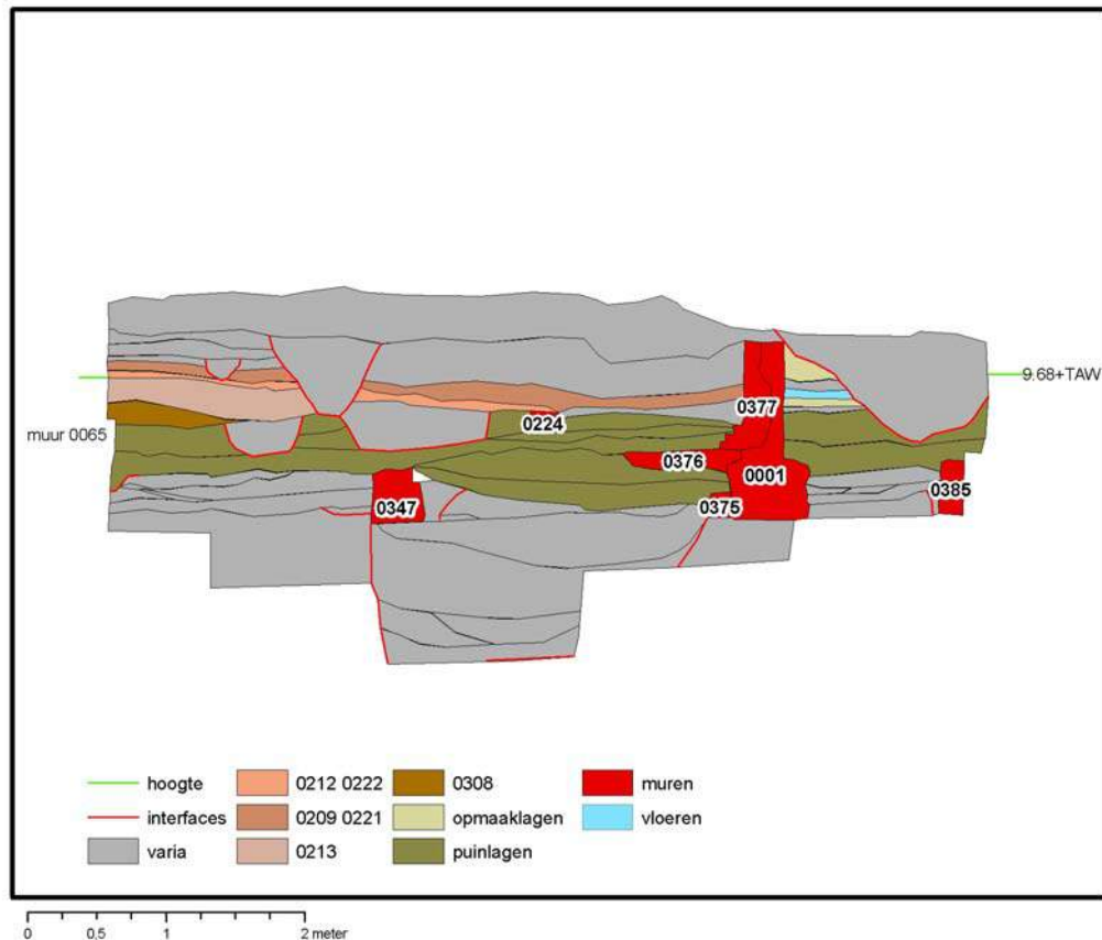
Figuur 3.3.5-199: profiel 2
