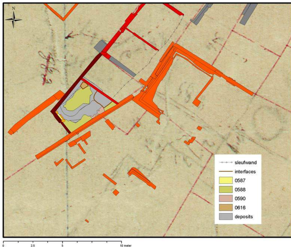
Figuur 3.3.7-65: uitbreiding achterhuis, met in het donkerrood muren 0584 en 0585 en in het geel schouw 0586.
