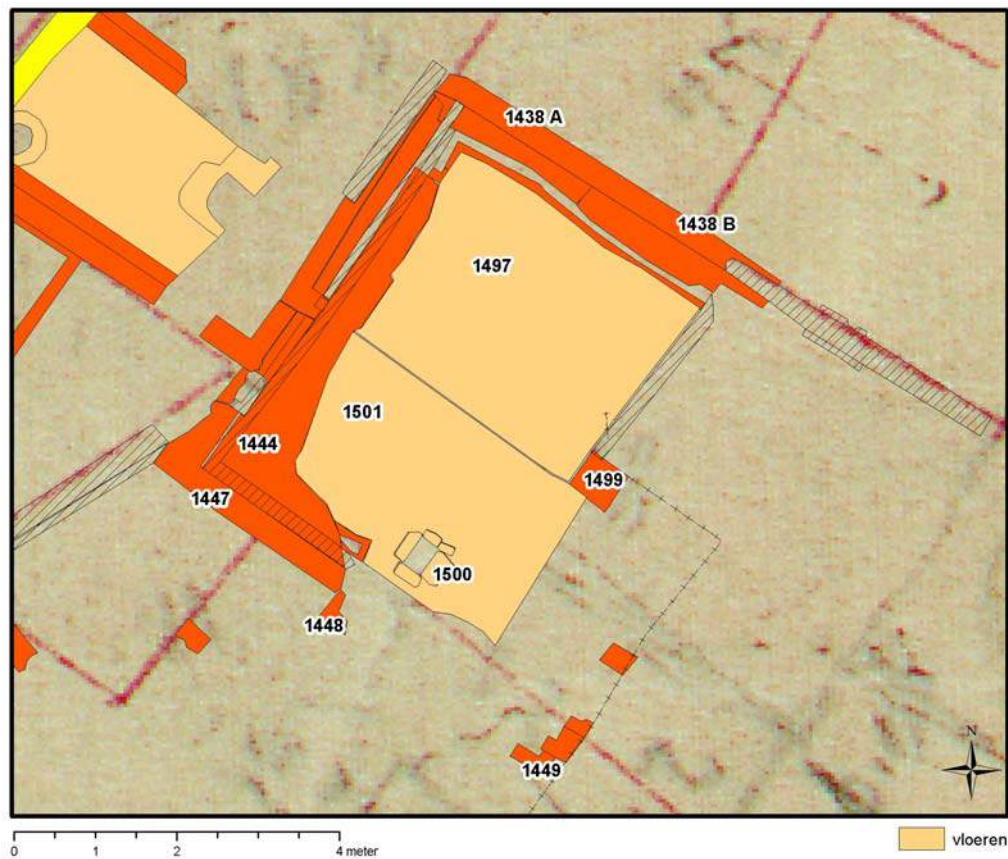
Figuur 3.3.5-151: keldervloer
