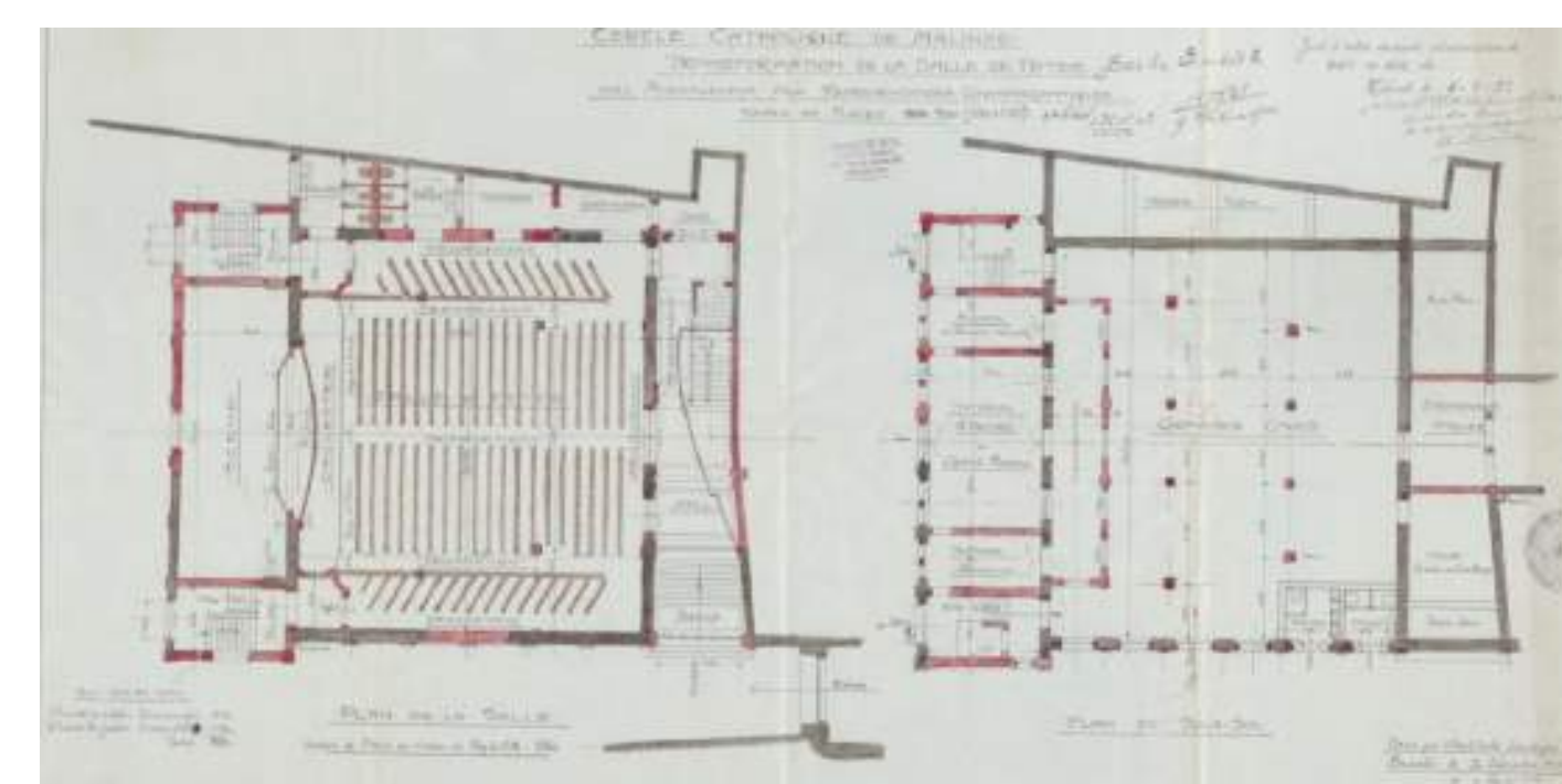
©Stadsarchief Mechelen • Bouwplannen van Het Volksbelang, nu gekend als het TheAtrium
